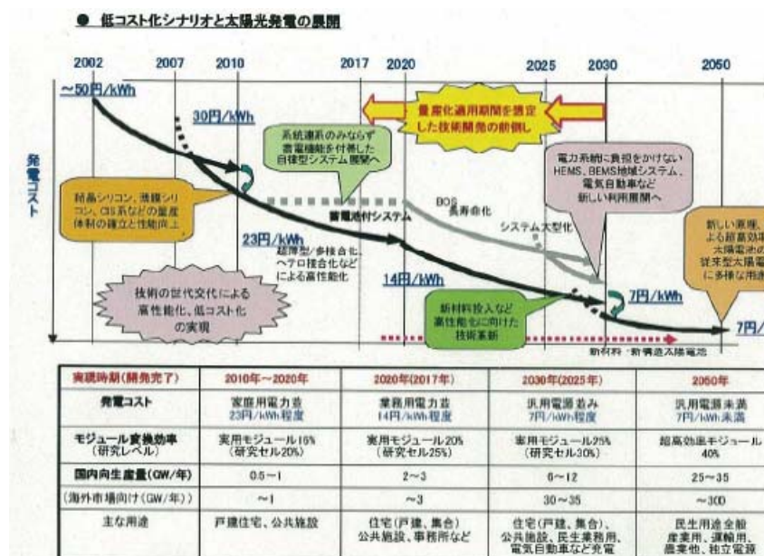
図2 太陽光発電の今後の発展に対するロードマップ(PV2030+)のシナリオ
